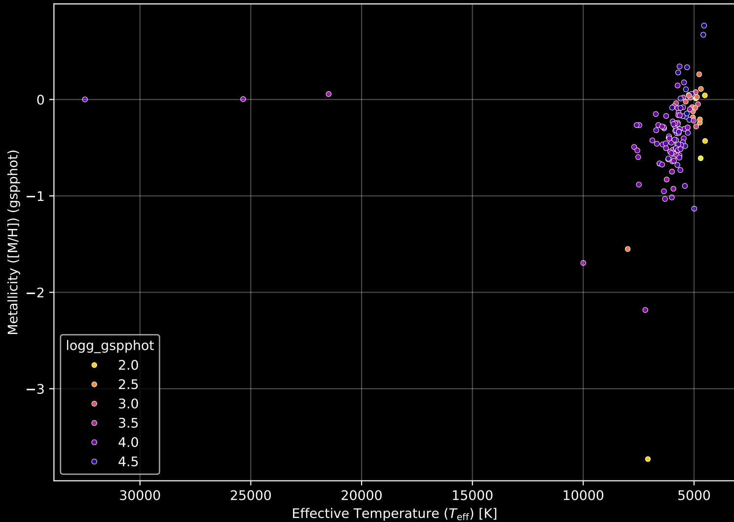
GALAH DR4 Field: [7177] Stellar Population Parameters (n= 130)
